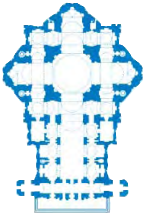
Plan de la Basilique Vaticane – Période Baroque.
